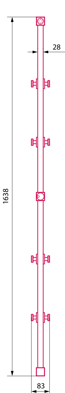
Вид спереди
