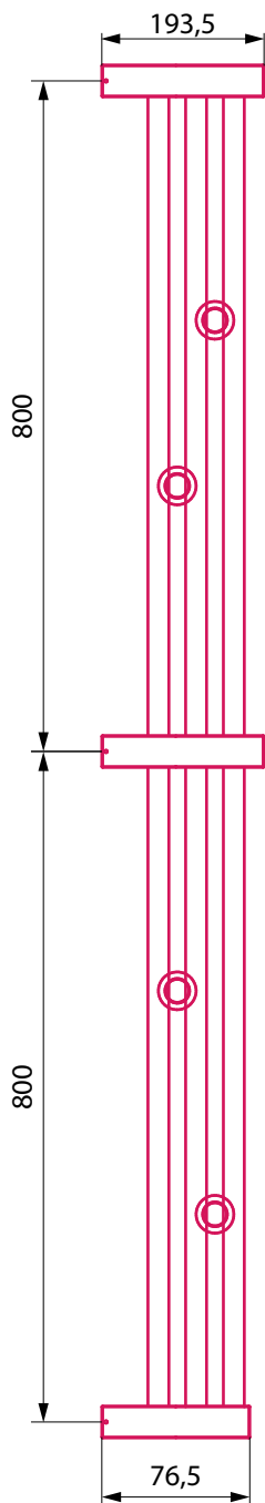
Вид сбоку
