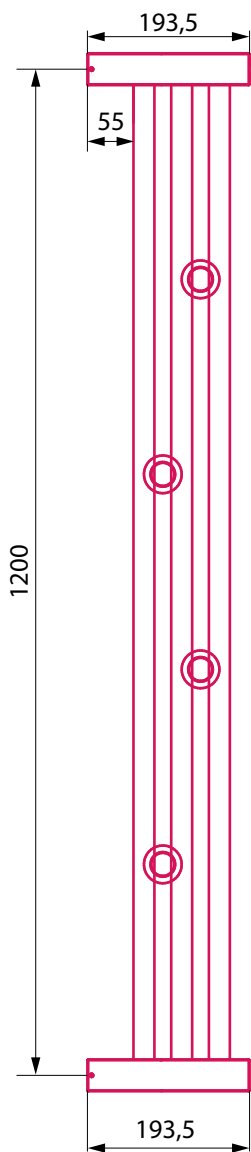
Вид сбоку
