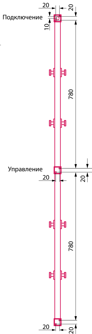
Вид сзади
