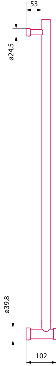
Вид сбоку
