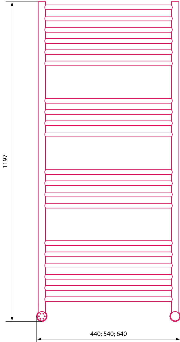
Вид спереди
