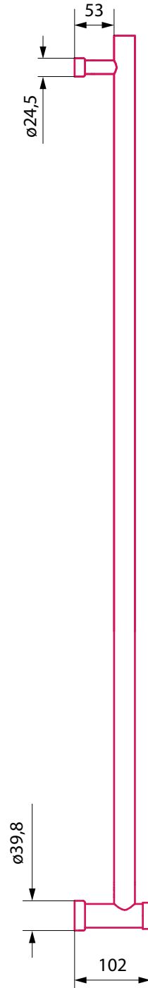
Вид сбоку
