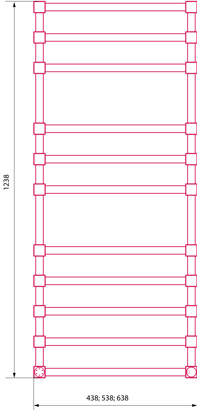
Вид спереди
