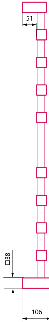
Вид сбоку
