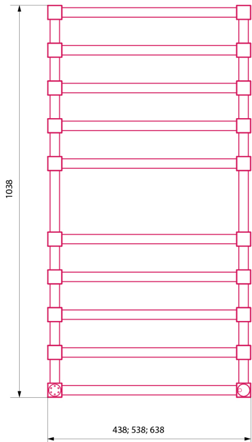
Вид спереди
