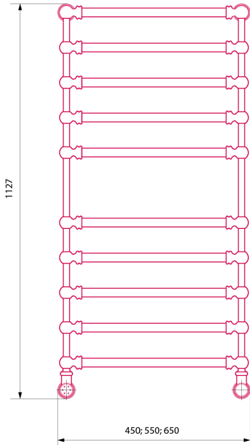
Вид спереди
