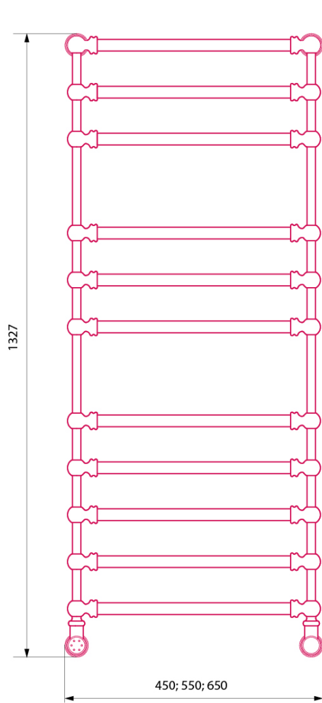
Вид спереди
