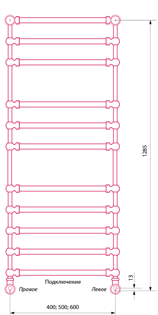
Вид сзади
